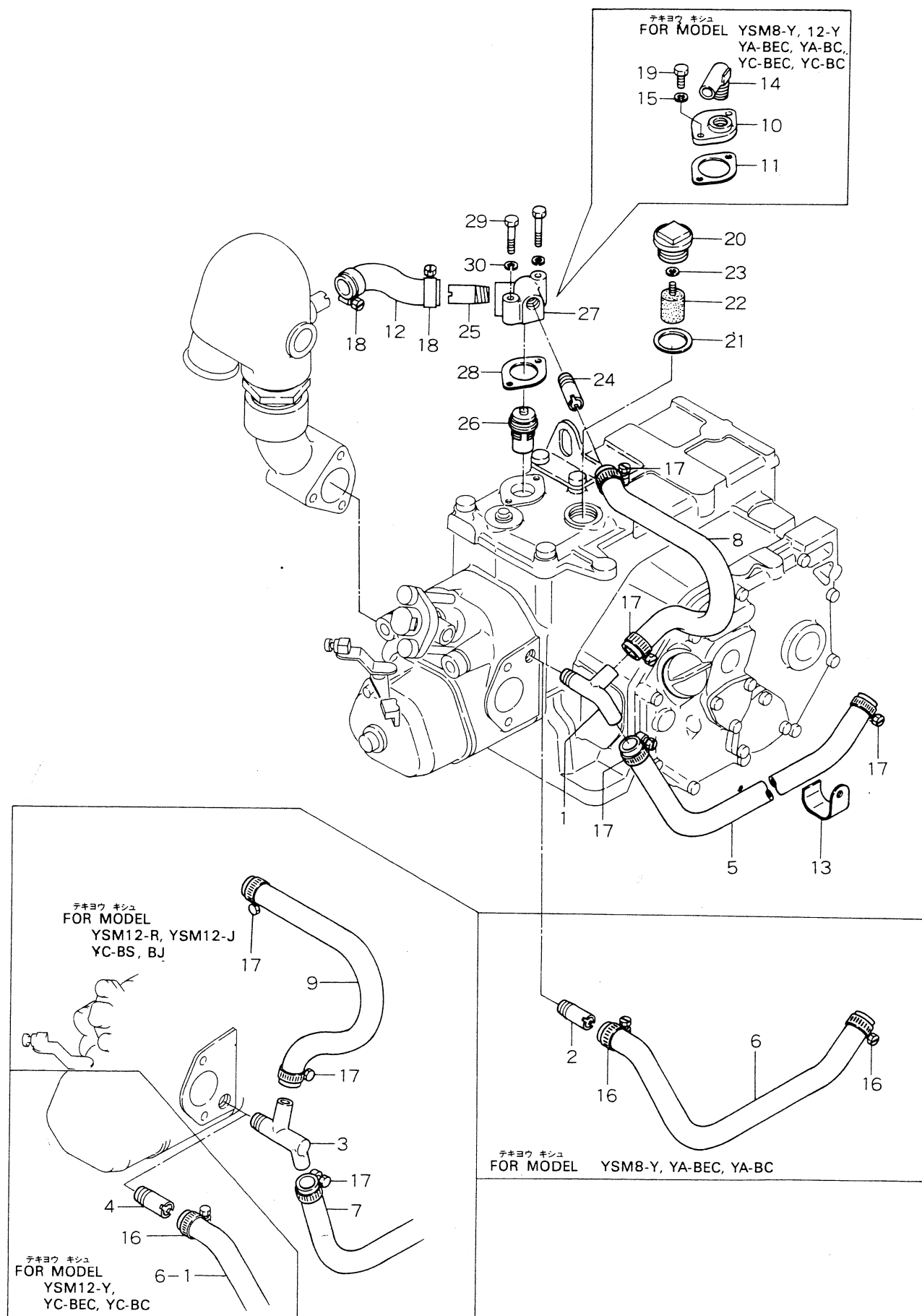
クーリング ウォータ システム Fig. 9 COOLING WATER SYSTEM
