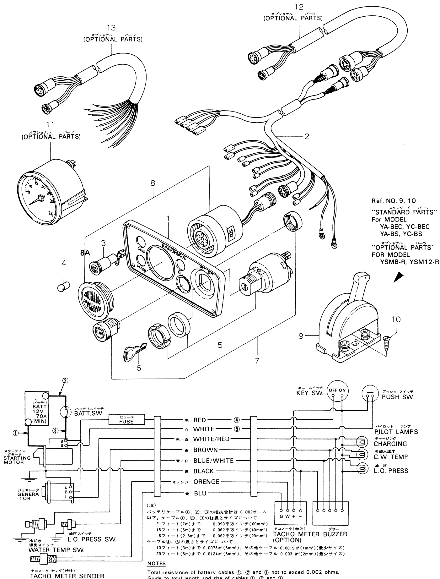
インストルメント パネル Fig. 17 INSTRUMENT PANEL
