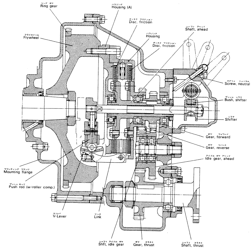
クラッチ セクショナル ビュー Fig. 18 CLUTCH SECTIONAL VIEW
